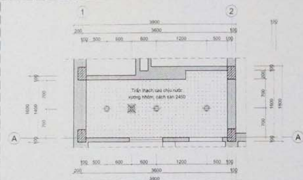
MẶT BẰNG TRẦN WC1
