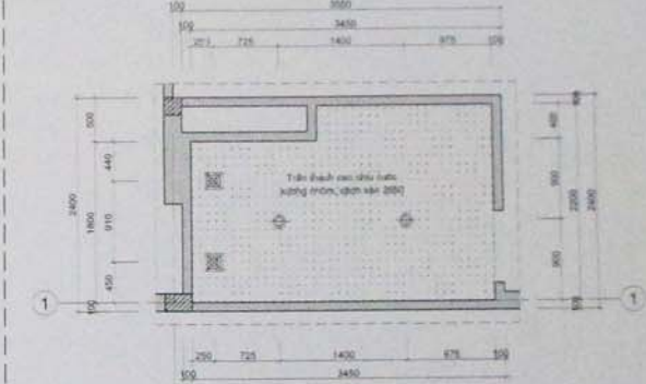
MẶT BẰNG TRẦN WC2
