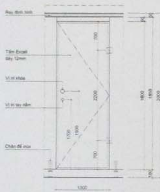
CHI TIẾT VÁCH NGĂN
