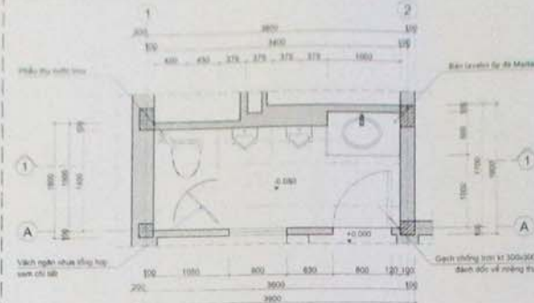
MẶT BẰNG WC1
