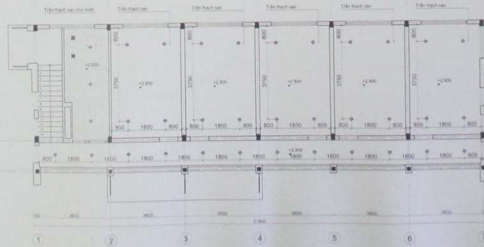
MẶT BẰNG TRẦN TẦNG 2
